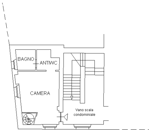
PIANO PRIMO H=3,10 ml
